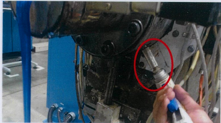
Bước 5: Sử dụng súng bắn khí xịt thẳng vào trong lỗ khí để gèn đi ra ngoài
